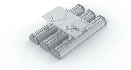
V4-10-70.0004.IRO-0001 Подвесное крепление для 3 светильников Размер крепления 385x123x276мм
