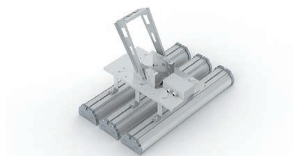
V4-10-70.0002.IRO-0002 Поворотное крепление для 3 светильников Размер крепления 385x362x276мм (при положении скобы перпендикулярно светильникам) Угол поворота 180°, шаг 15°
