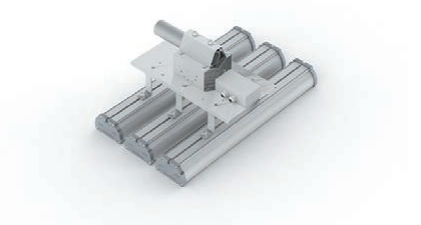
V4-10-70.0003.IRO-0001 Консольное крепление для 3 светильников Размер крепления 385x220x276мм Установка на консоль диаметром 40÷50мм
